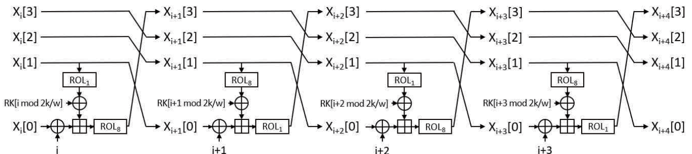
(그림 2) CHAM의 라운드 함수
