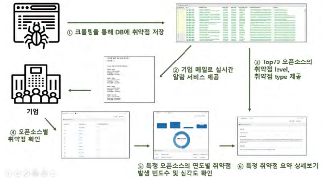
그림 1 동작 흐름도
