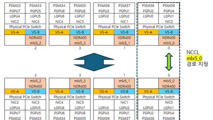
(그림 3) NCCL PXN 활성화 구성도
