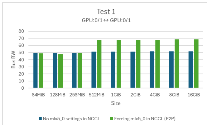
<표 1> Forcing mlx5_0 (P2P) 사용 전 후 Bandwidth 비교
