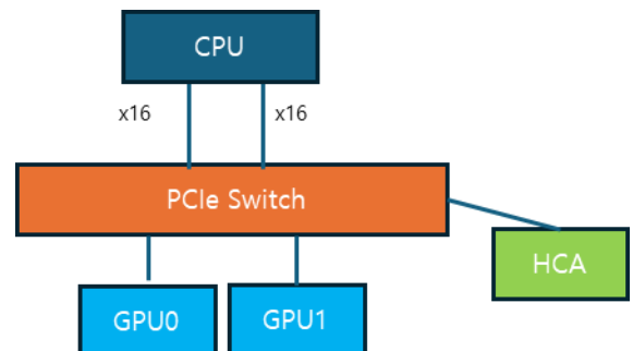
&lt;그림 4&gt; CPU↔GPU↔NIC 경로 관계
