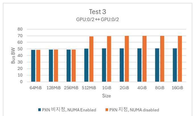
<표 3> BIOS 최적화 전, 후 Bandwidth 비교
