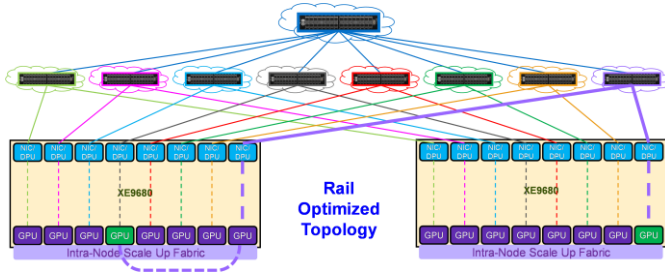
(그림 2) Rail Optimized 구성도
