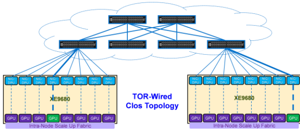
(그림 1) Clos Topology 구성도 사진
