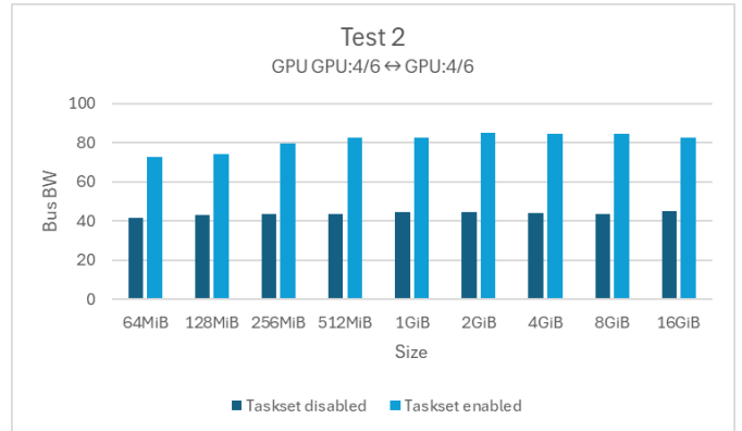
<표 2> CPU Affinity 사용 전, 후 Bandwidth 비교
