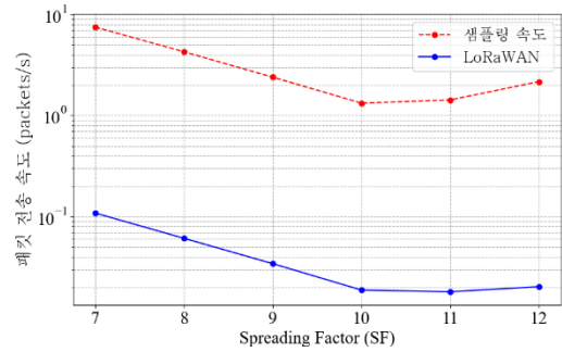
(그림 2) 샘플링 속도와 LoRaWAN 의 패킷 전송 속도 비교. 센싱에 요구되는 속도가 LoRaWAN 에서의 속도보다 100 배 이상 높음.
