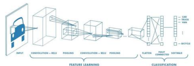
(그림 1. CNN 기본 구조)
