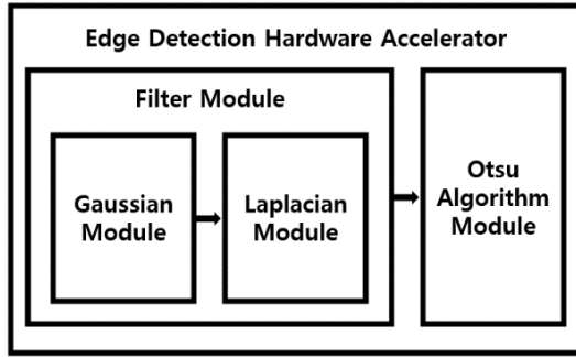
(그림 1) 엣지 검출 하드웨어 가속기 블록도
