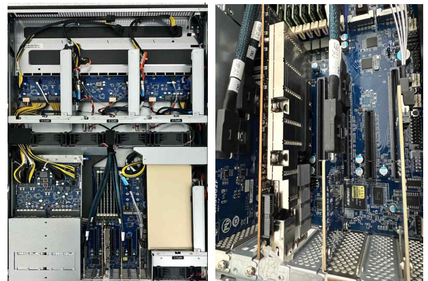
그림 5 BlueField DPU 테스트베드
