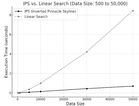
(그림 1) IPS와 선형 탐색 구동 시간 비교
