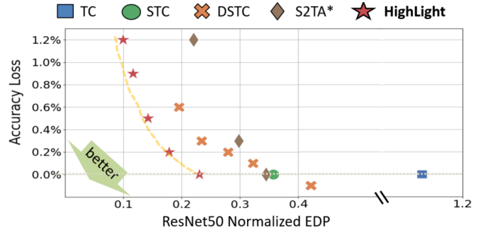
(그림 1) HighLight 의 EDP-정확도 성능 비교[7]
