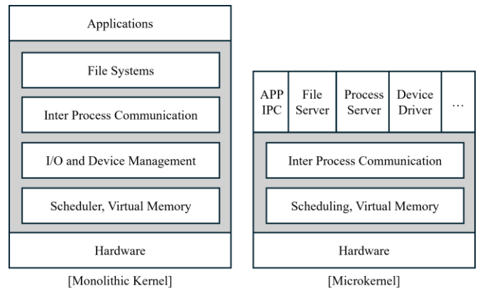
(그림 1) 모놀리식 커널과 마이크로 커널
