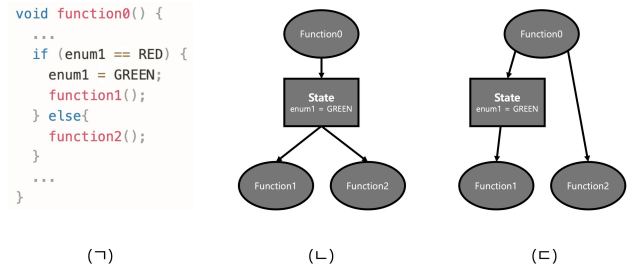
(그림 3) (가): 상태 전이가 일어나는 코드, (나): CG를 이용해 생성한 (가)의 상태 기계, (다): CG와 ICFG를 모두 고려해 생성한 (가)의 상태 기계
