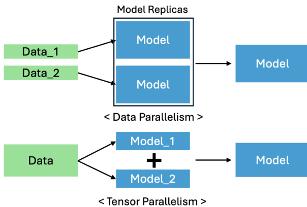
(그림 1) Data Parallelism 과 Tensor Parallelism
