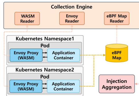
(그림 3) Collection Engine 동작도
