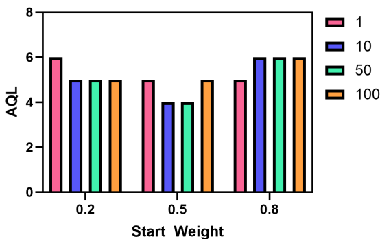
(그림 6) Average Queue Length(AQL)
