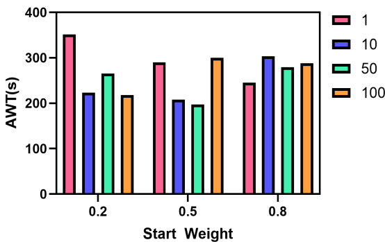
(그림 7) Average Waiting Time(AWT)
