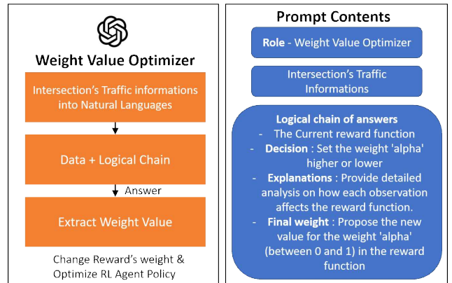
(그림 4) LLM 구조와 프롬프트 내용
