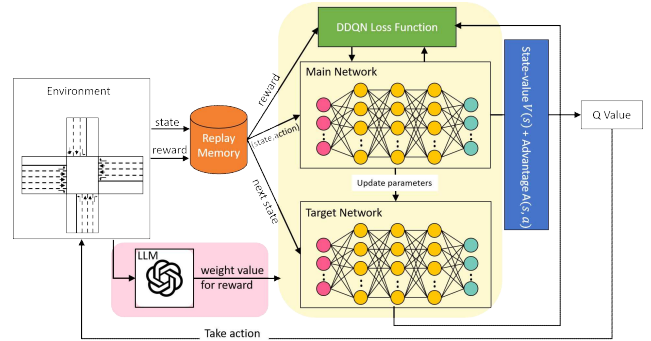
(그림 2) D3QN-LLM 프레임워크
