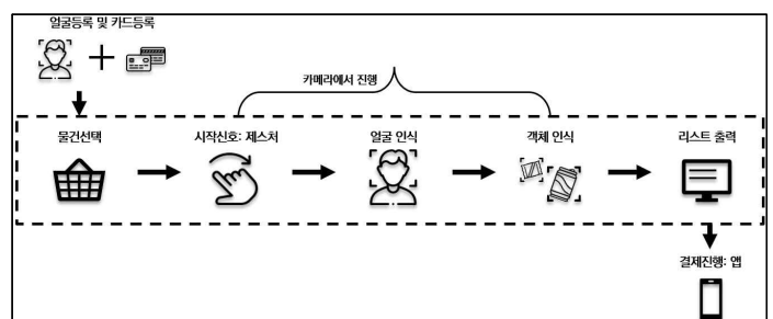
그림 1. 시나리오 흐름
