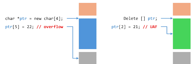
(그림 1) ARM MTE의 동작 방식
