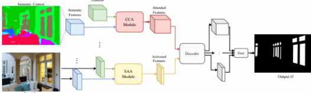
그림 2 GlassSemNet 시스템 모델 예시
