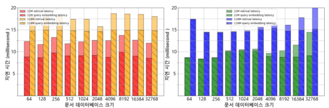
(그림 5) 모델 크기 별 쿼리 임베딩, 검색속도 실행시간 변화(데이터베이스 종류-좌:Chroma, 우:FAISS)
