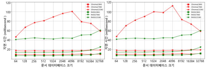
같은 사이즈의 임베딩 모델의 비교
