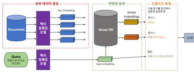
(그림 1) RAG 실행 과정
