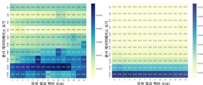
(그림 2) 조건별 지연 시간 비교 (좌: Chroma, 우: FAISS)
