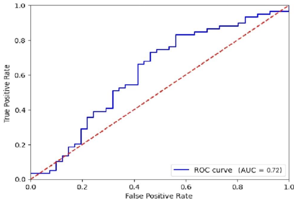
(그림 2) 훈련된 모델의 ROC Curve
