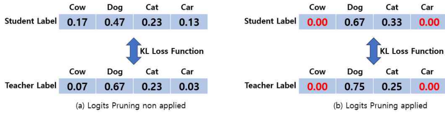
(그림 2) Logits Pruning의 적용 방법 도식화, (a)와 (b)는 Logit Pruning 적용 전, 후를 표현
