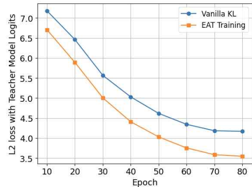
(그림 3) Vanilla 지식 증류 기법과 EAT 기법을 적용했을 때의 L2 Loss 변화 차이
