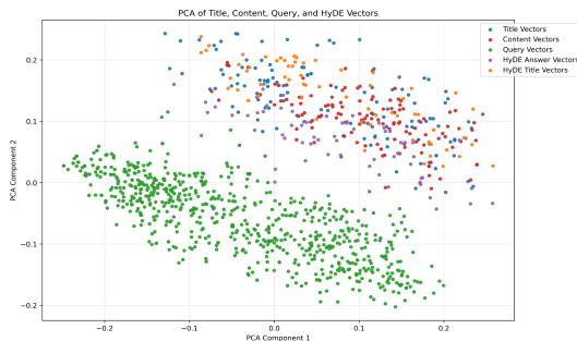
그림 2. 임베딩 벡터 PCA 시각화
