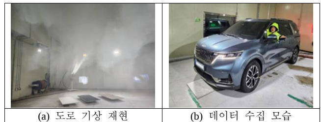
(그림 4) 도로 기상 재현 및 음파 데이터 수집 환경
