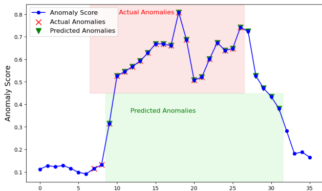
(그림 2) TKAD 모델의 집합적 이상 탐지
