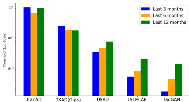
(그림 3) 학습 기간에 따른 모델별 최적 임계값
