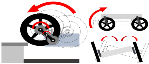
(그림 1) 편심 메커니즘 이용 단차 극복, 기울기 조절
