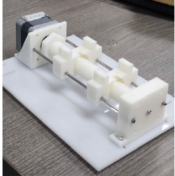
(그림 3) 너트에 구조물을 덧대어 너트가 볼트에 수직으로 고정된 모습
