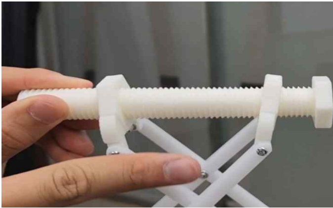
(그림 2) 너트가 볼트에 수직으로 고정되지 않아 비틀어진 모습
