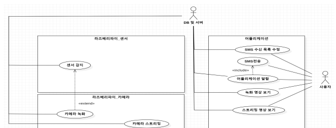
그림 1 . 유스케이스 다이어그램
