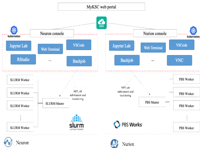
(그림 1) MyKSC 아키텍처
