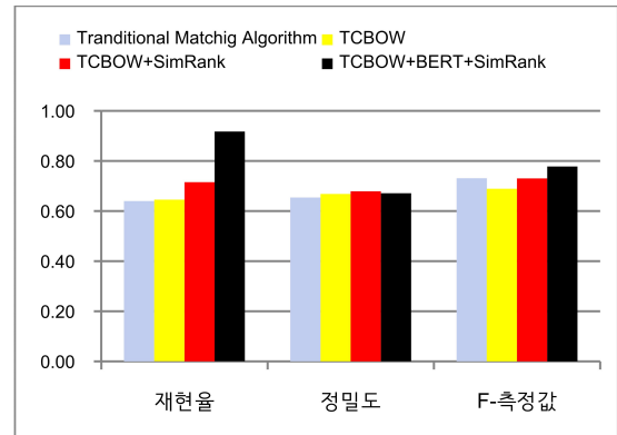
(그림 3) FMA-SNOMED 데이터셋 결과
