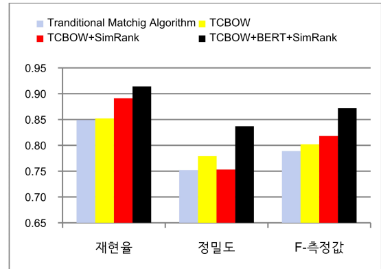
(그림 2) FMA-NCIT 데이터셋 결과
