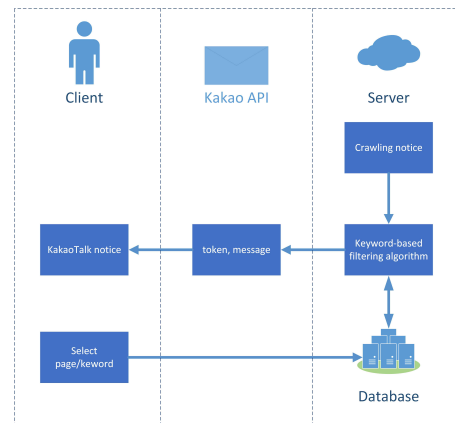
(그림 1) 제안된 웹 크롤링 기반의 개인 맞춤형 정보제공 앱 서비스의 흐름도
