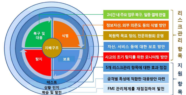
(그림 2) CPMI-IOSCO 사이버복원력 체계 개요
