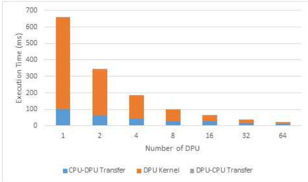
그림 4 강화장성 성능 분석 (SR, Total Points = 4,096,000)
