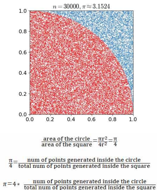
그림 2 몬테카를로 원주율 추정
