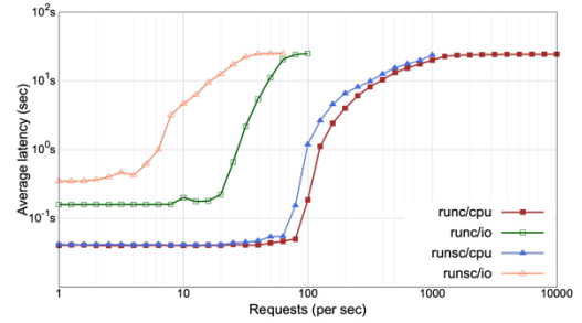
(그림 3) 런타임별 요청 횟수에 따른 평균 응답 시간
