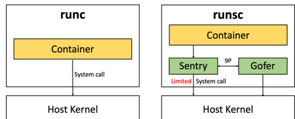
(그림 1) runc 와 runsc 구조
