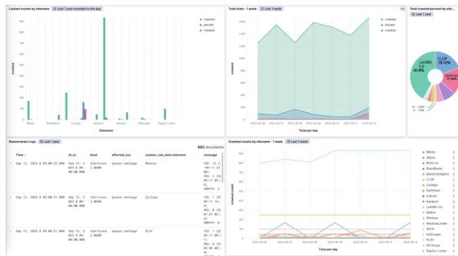
(그림 2) 랜섬웨어 데이터 모니터링 Kibana 대시보드.
