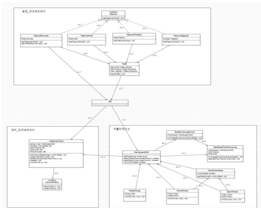
(그림 2) 클래스 다이어그램.
