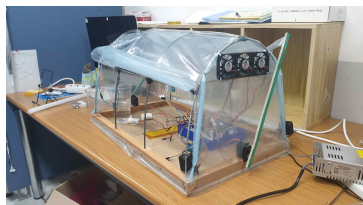
(그림 3) 라즈베리파이로 구현한 축소모형의 온실
