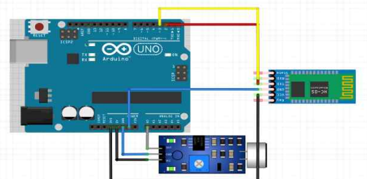
그림 2. 아두이노 회로도
