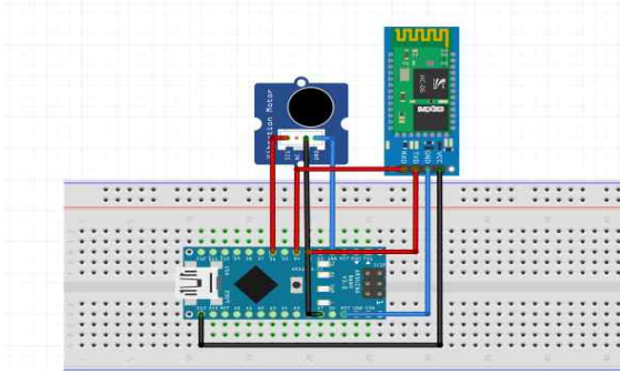
그림 3. 아두이노 회로도 2
