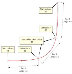
그림 1. 좌회전 궤적의 구성
