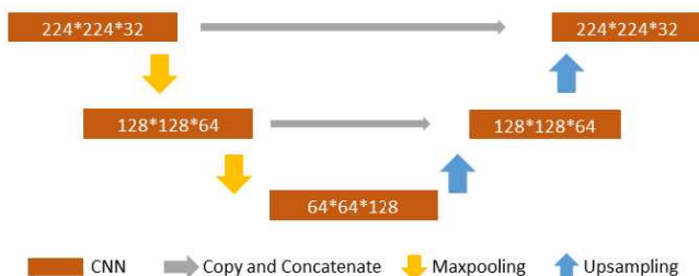
(그림 1) U-Net 구조를 가진 신경망의 예시.
