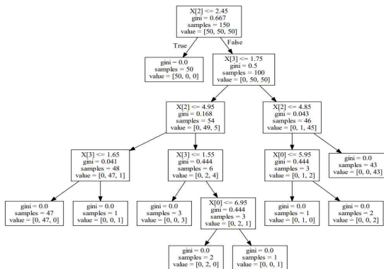
(그림 1) 의사결정나무 도식화 예제
