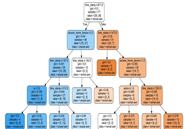
(그림 2) 구현된 의사결정나무 도식화
