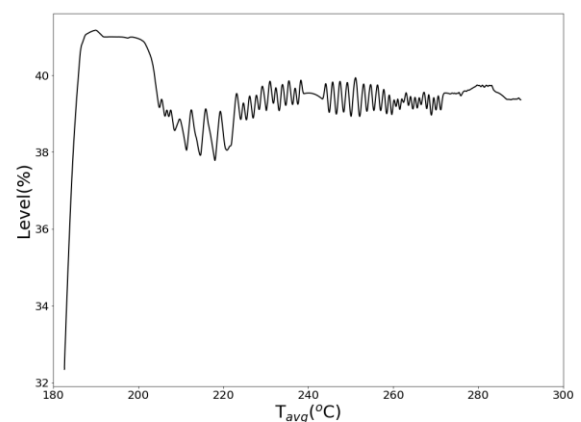
(그림 5) 실험결과 - 가압기 수위 제어
