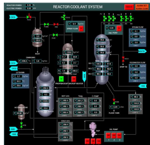
(그림 1) compact nuclear simulator 화면
