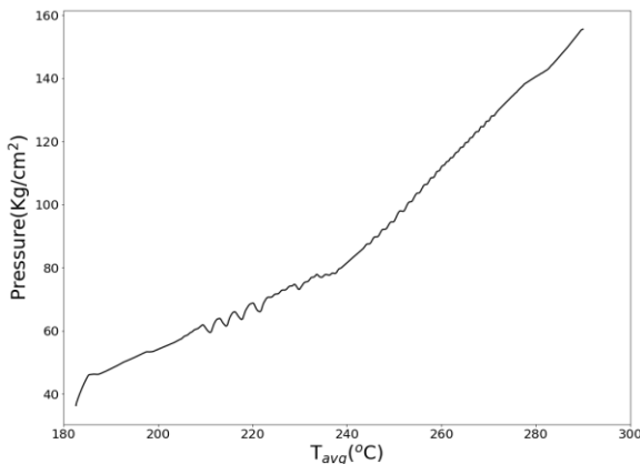
(그림 6) 실험결과 - 가압기 압력 제어
