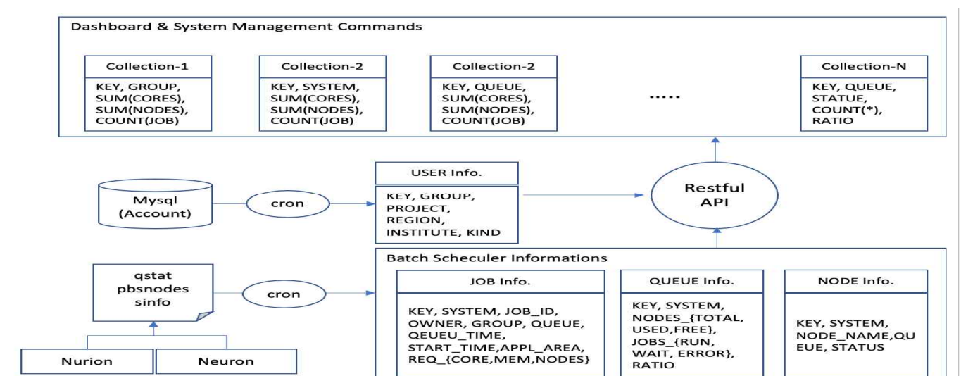
<그림 3> 데이터 흐름도
