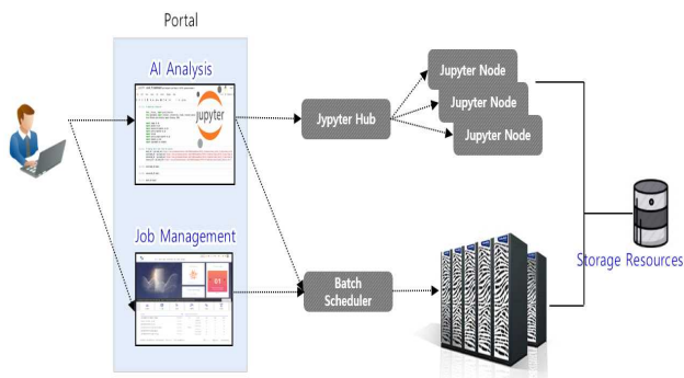
<그림1> 특징 데이터 추출 자동화 시스템 구성도
