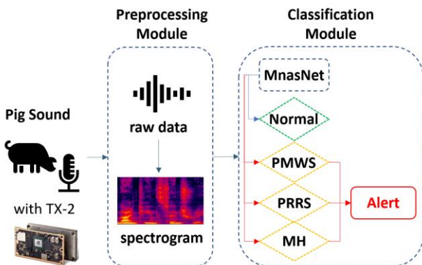
(그림 1) 소리 신호를 이용한 경량 딥러닝 기반의 돼지 호흡기 질병 탐지 시스템
