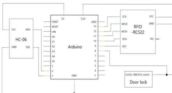
(그림 3) 도어록과 결합한 아두이노 회로도
