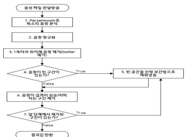
[그림 6] 음성분석 알고리즘 순서도
