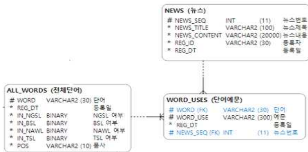
[그림 3] 엔티티 관계도
