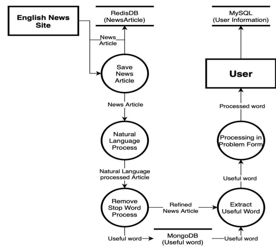
[그림 2] 데이터의 흐름 및 절차도
