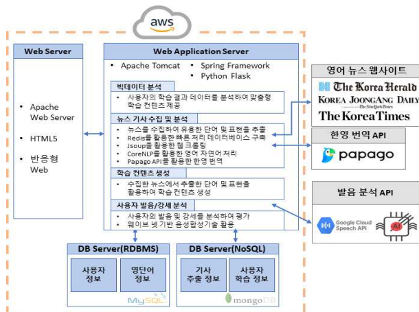
[그림 1] 빅데이터 영어학습 시스템 구성도
