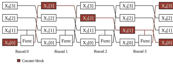
(그림 4) CHAM 카운터 운용 모드의 구조
