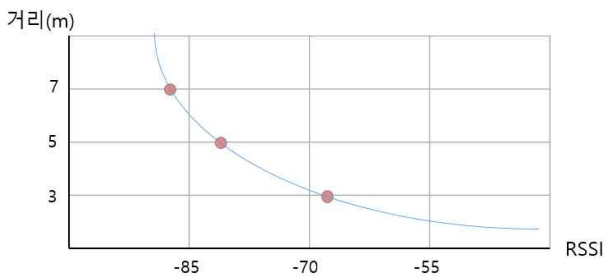
(그림 8) 스플라인 보간법 다차원 방정식 예제
