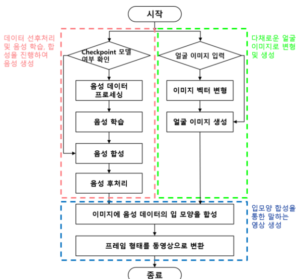
(그림 2) AI 아나운서의 시스템 흐름도
