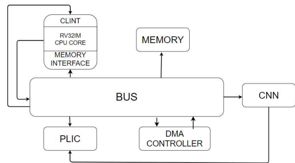
(그림 3) RISC-V VP 모듈 구조도
