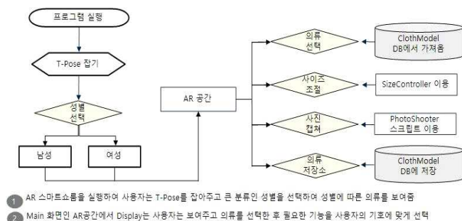
그림 7 기능 흐름도
